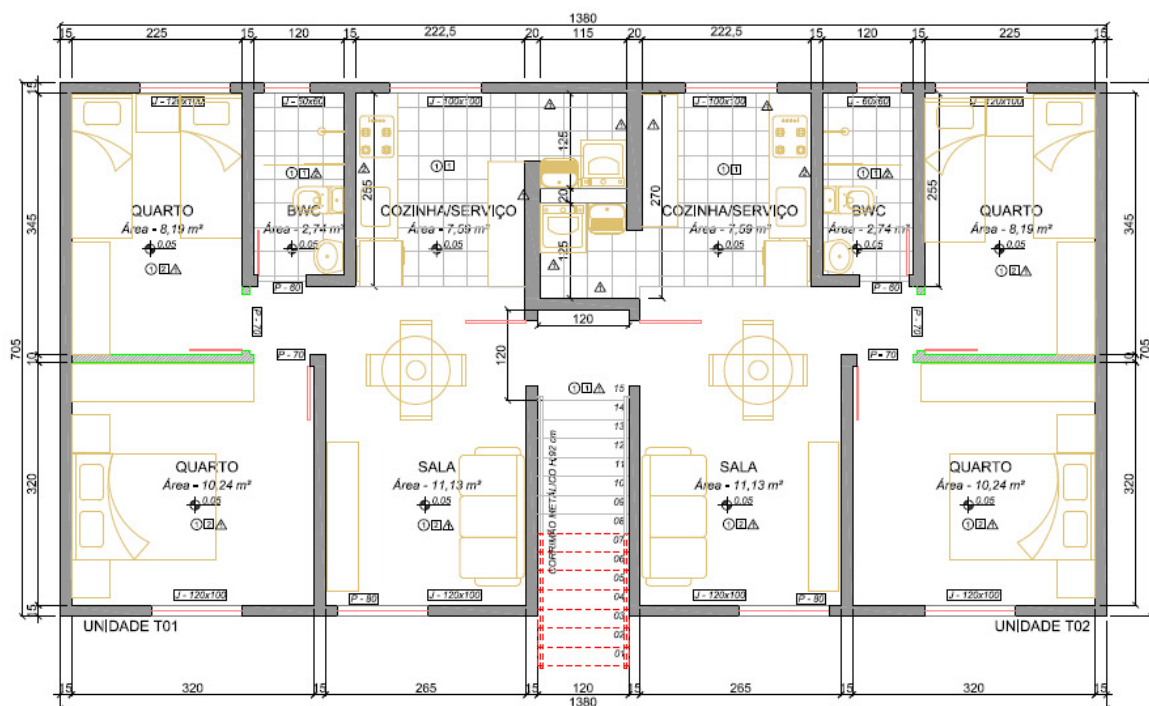
Figura 8: Planta baixa do pavimento superior
