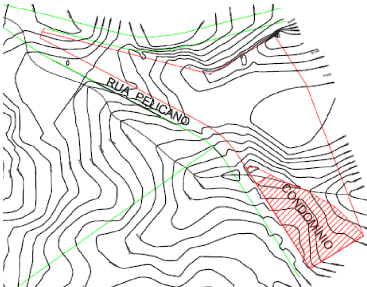
Figura 9: Levantamento planialtimétrico
