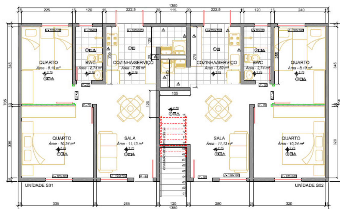
Figura 7: Planta baixa do pavimento térreo
